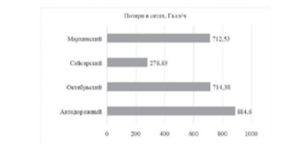
Рисунок 12 – Потери в сетях по энергорайонам АО «Теплоэнергия» в Гкал/ч
